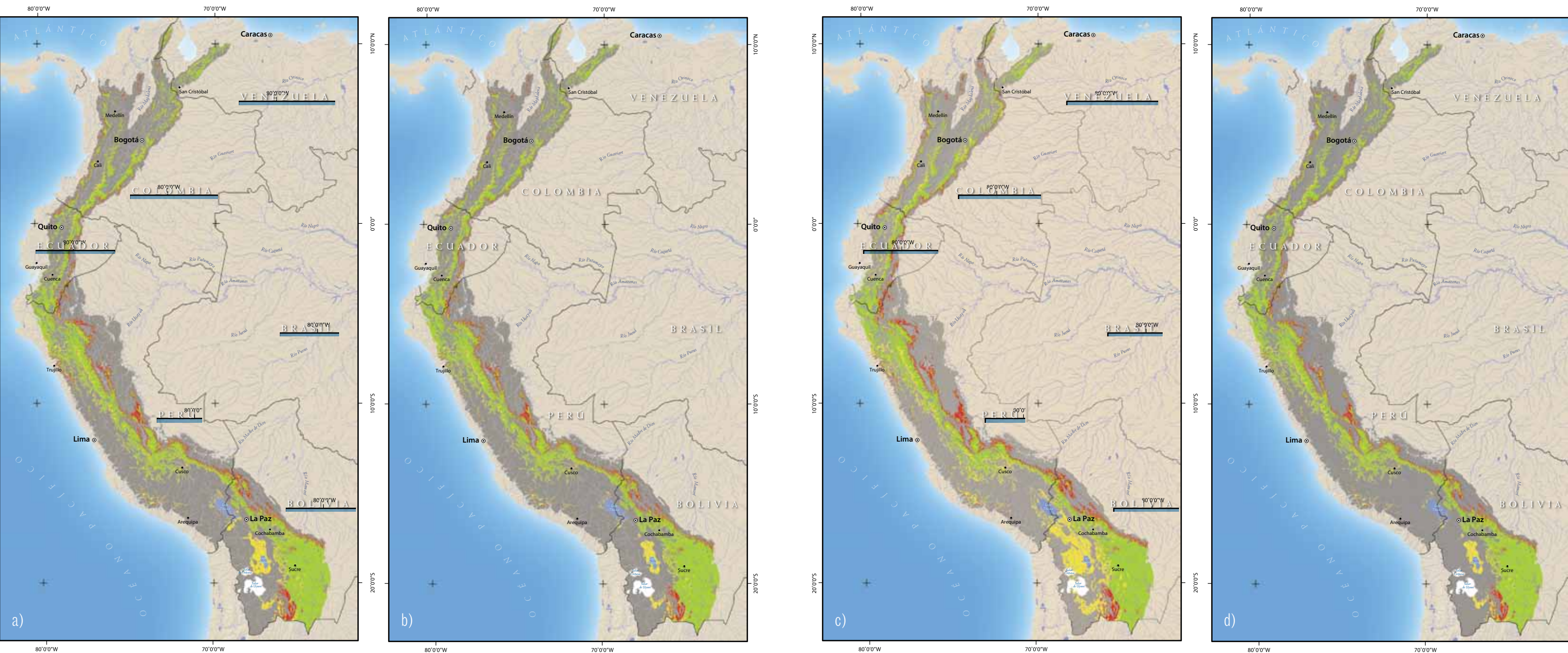
Figura 10. Patrones de áreas estables, pérdida y ganancia de bosques montanos, para distintos escenarios de cambio climático en el año 2050: a) CCMA A2; b) CCMA B2; c) HADCM3 A2, y d) HADCM3 B2.
